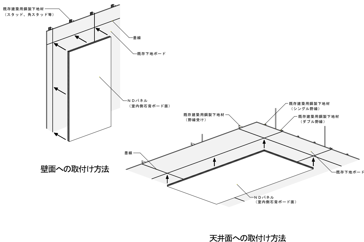
図3 壁、天井面への取付け方法
